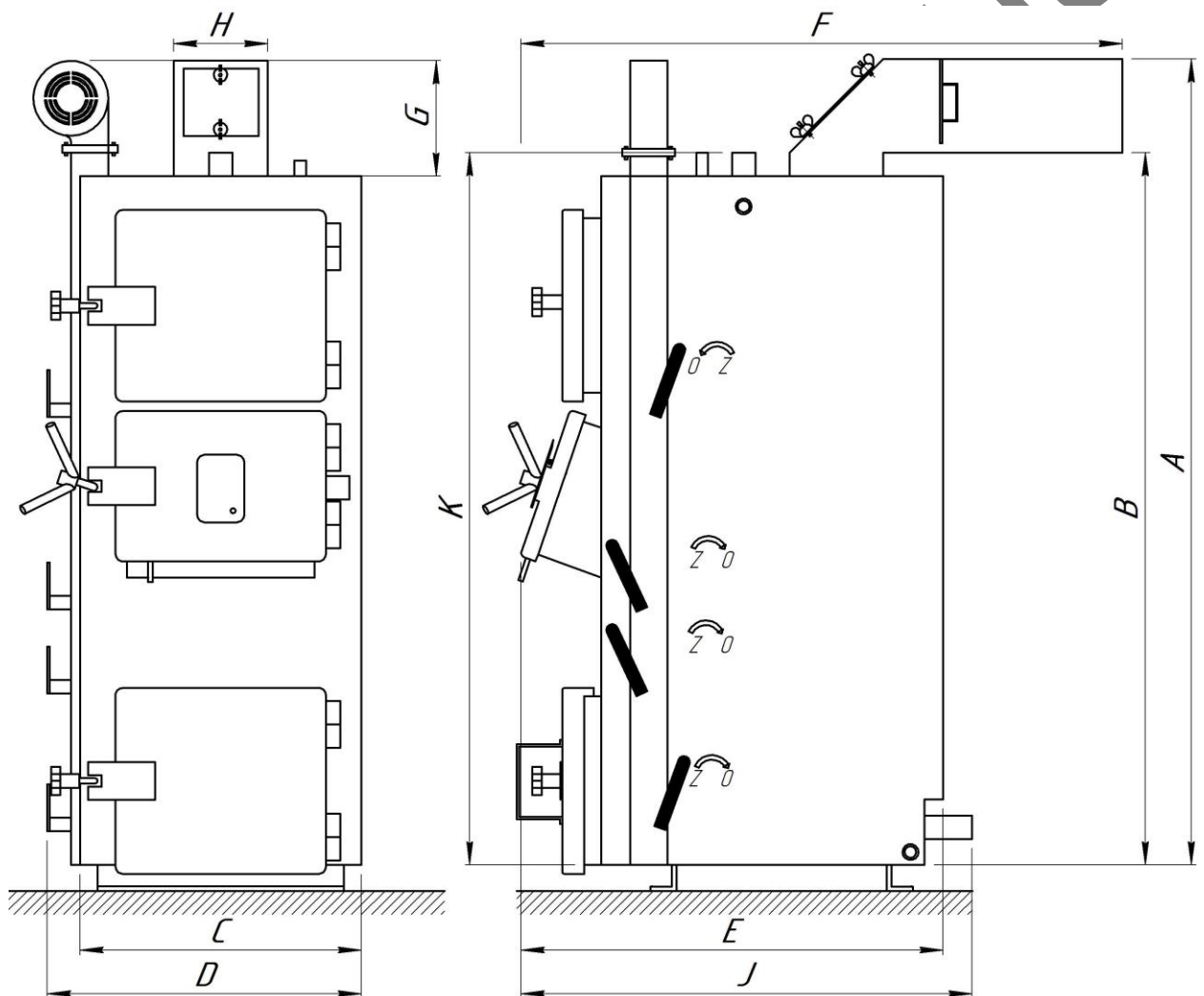
Рисунок 1 – Габаритне креслення котла типу LUX-1
